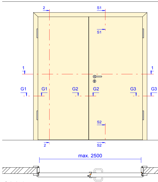
Schnitt 1
